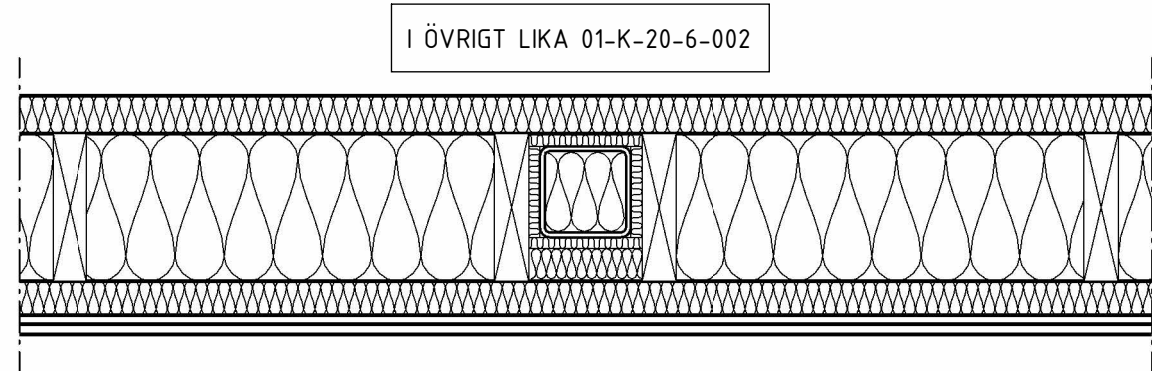
03 1 : 10 STÅLPELARE I FLÄKTRUMSVÄGG
