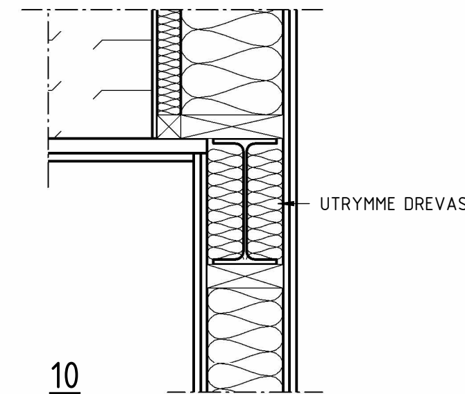
10 1 : 10 STÅLBALK I BÄRANDE INNERVÄGG
