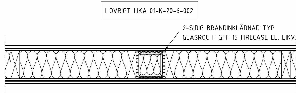
02 1 : 10 STÅLPELARE I BÄRANDE INNERVÄGG
