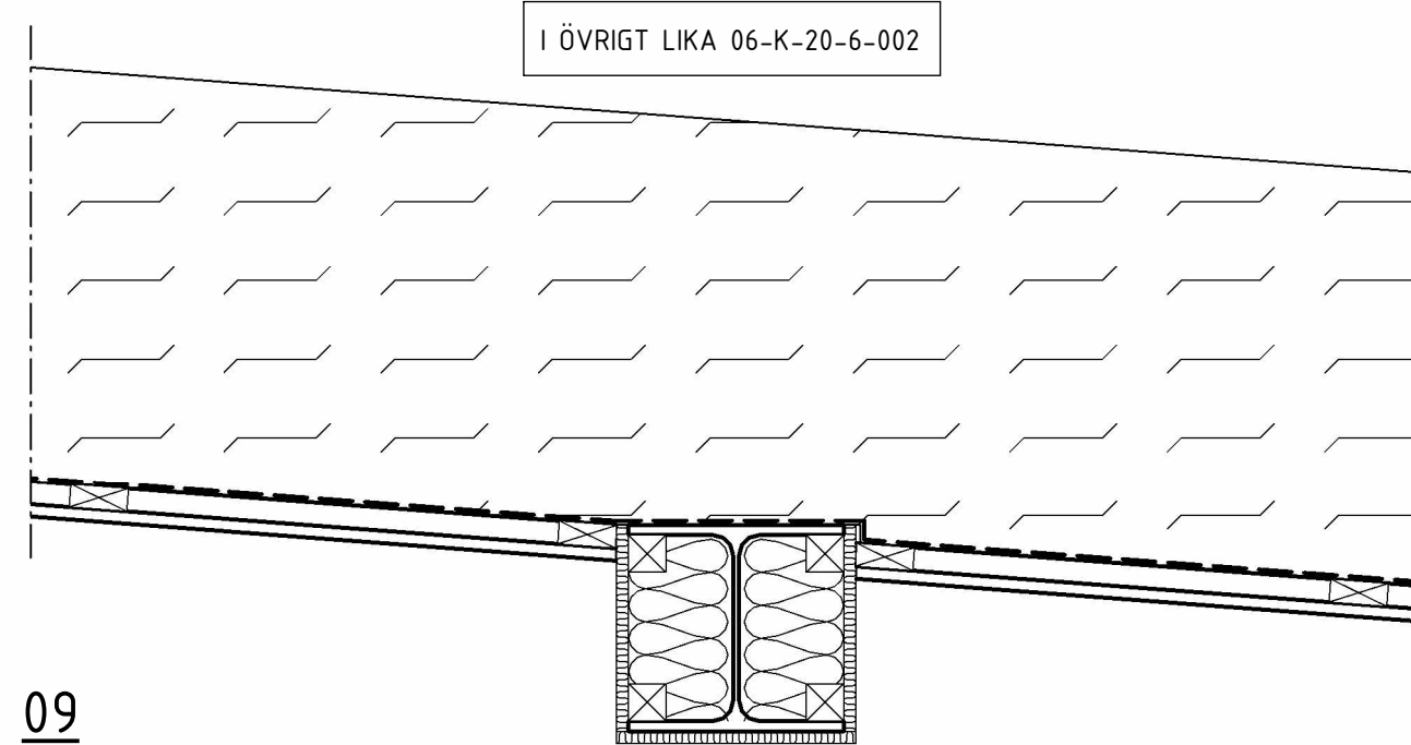
09 1 : 10 STÅLBALK UNDER TAKSTOLAR
