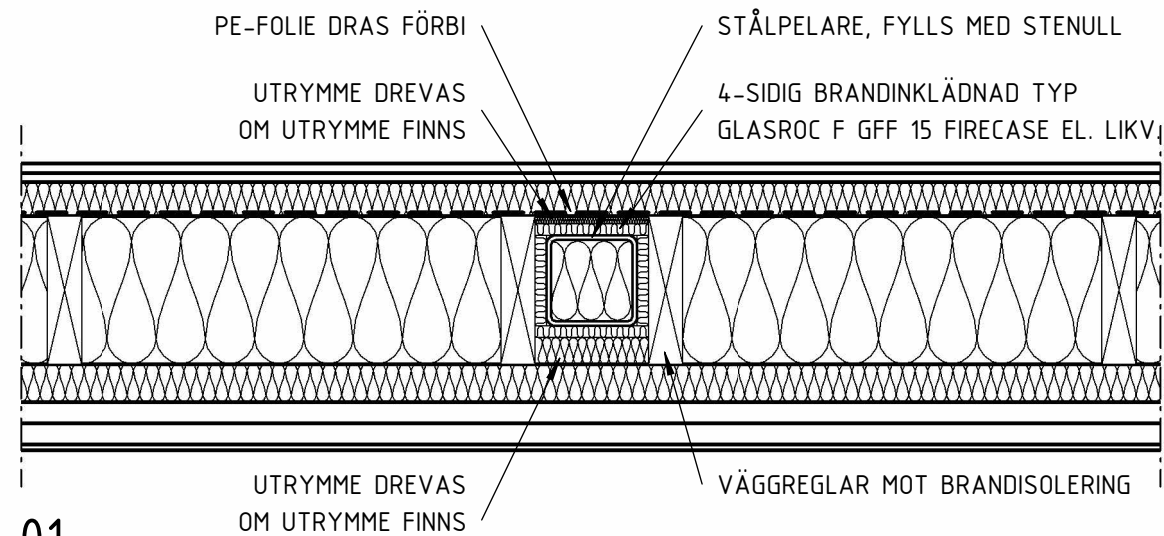
01 1 : 10 STÅLPELARE I YTTERVÄGG
