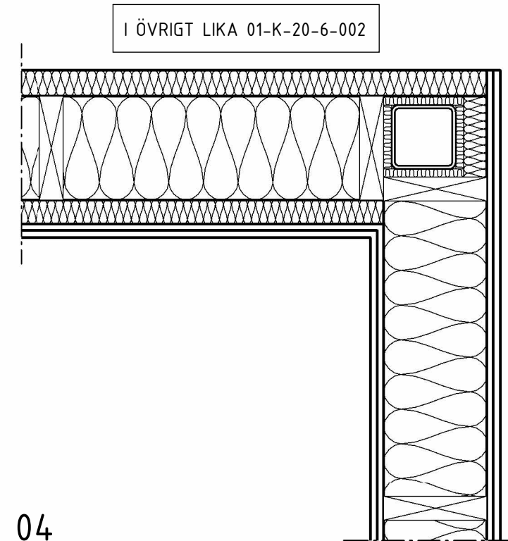
04 1 : 10 STÅLPELARE I FLÄKTRUMSVÄGG HÖRN
