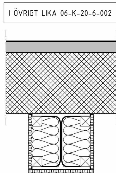
07 1 : 10 STÅLBALK UNDER HÅLDÄCK MITTEN
