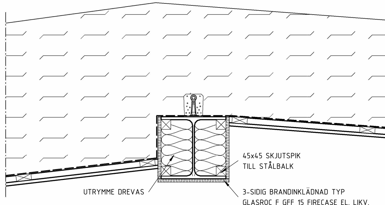
08 1 : 10 STÅLBALK UNDER TAKSTOLAR
